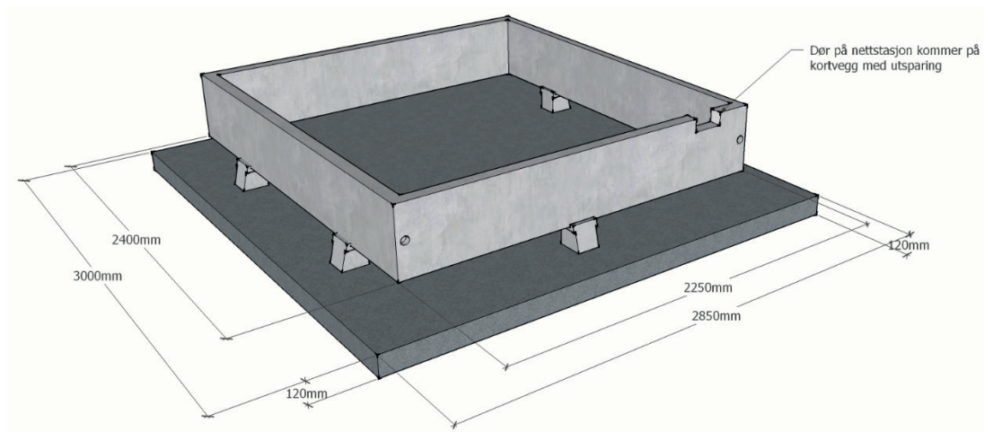
Figur 5. Fundament til prefabrikkert kiosk hvor fundamentet er 2400x2250 mm.
