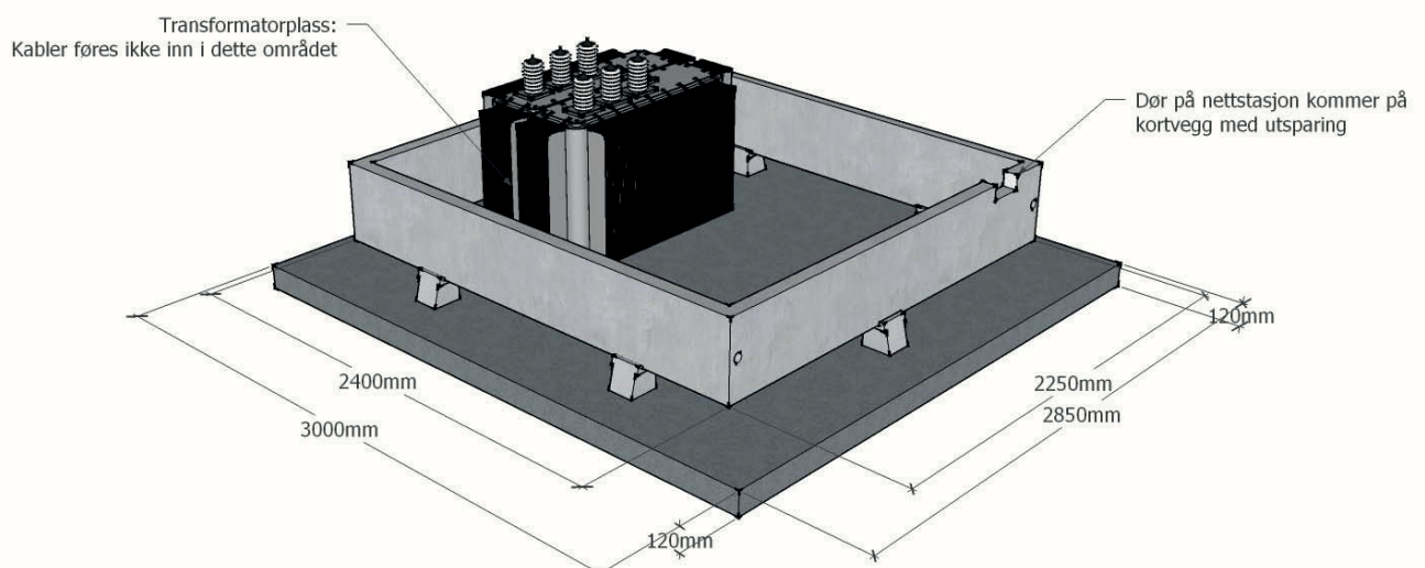
Figur 18. Innføring av kabler i prefabrikkert kiosk
