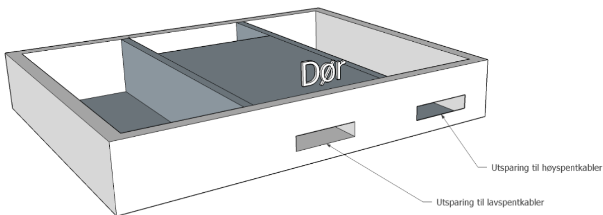
Figur 17. Innføring av kabler i ny betongnettstasjon
