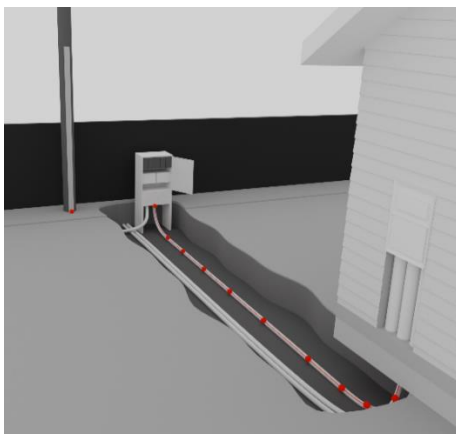
Figur 25-26 Innmåling av kabler.
