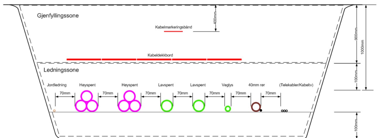
Figur 3. Grøftesnitt i veikryssing.
