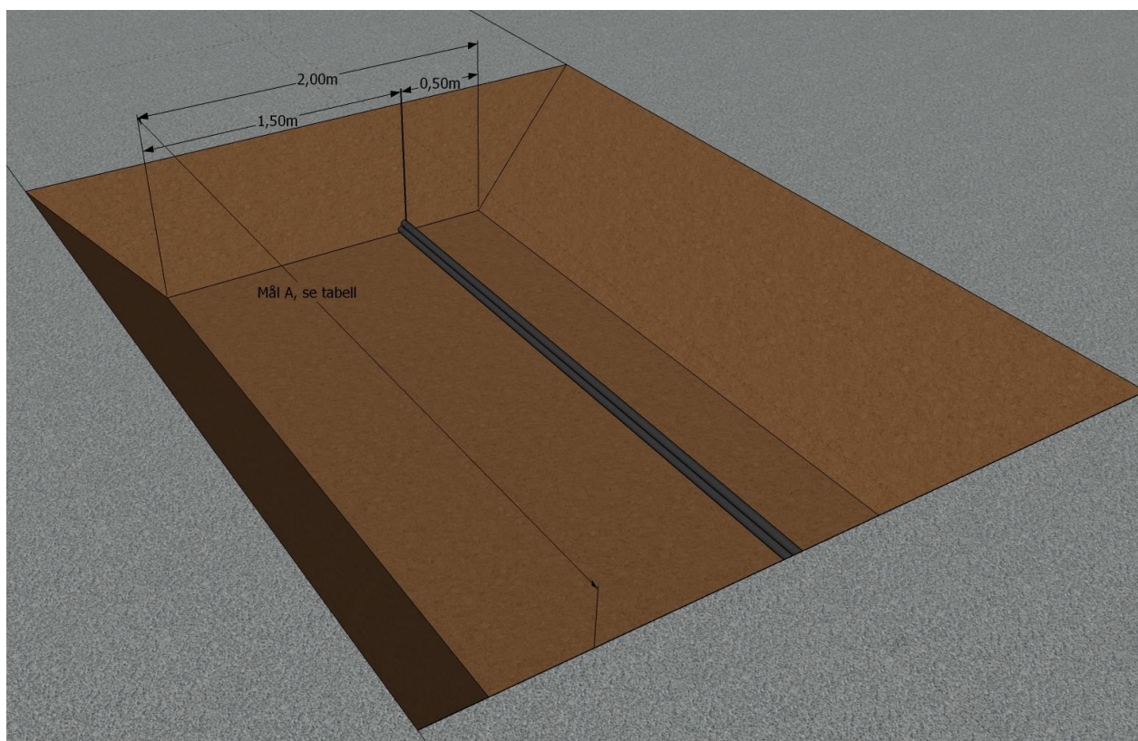
Figur 31. Skjøtegrøp
