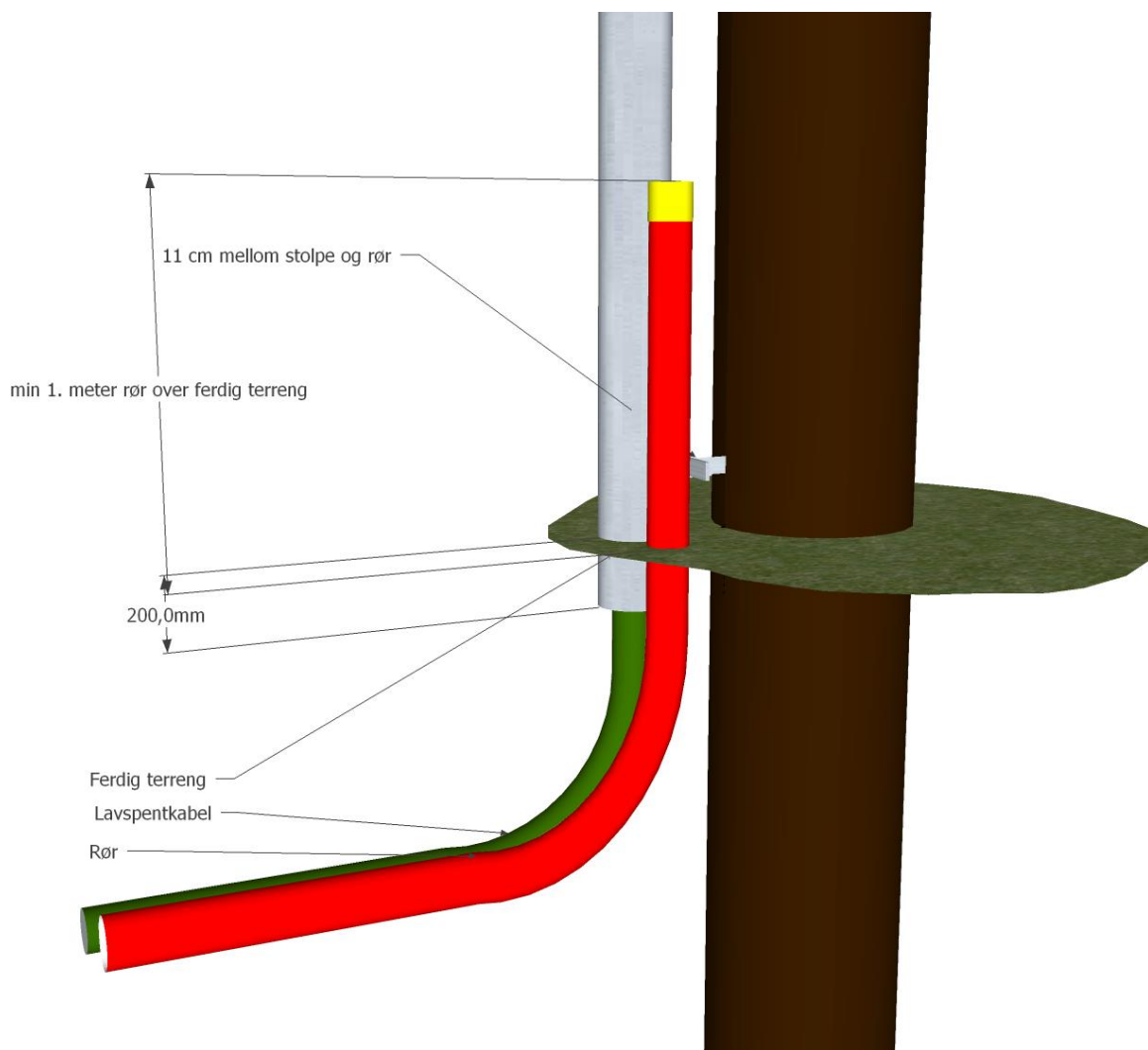
Figur 21 Oppføring av kabler og rør i mast
