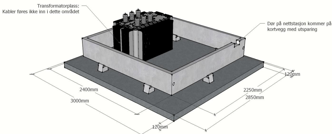
Figur 18. Innføring av kabler i prefabrikkert nettstasjon
