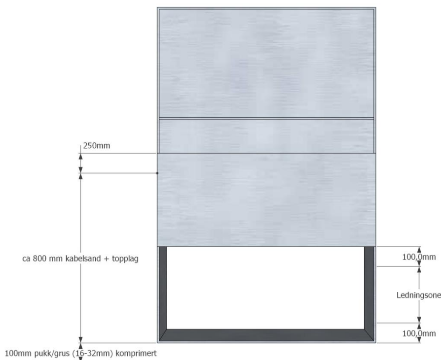
Figur 11. Fundamentering av kabelskap
