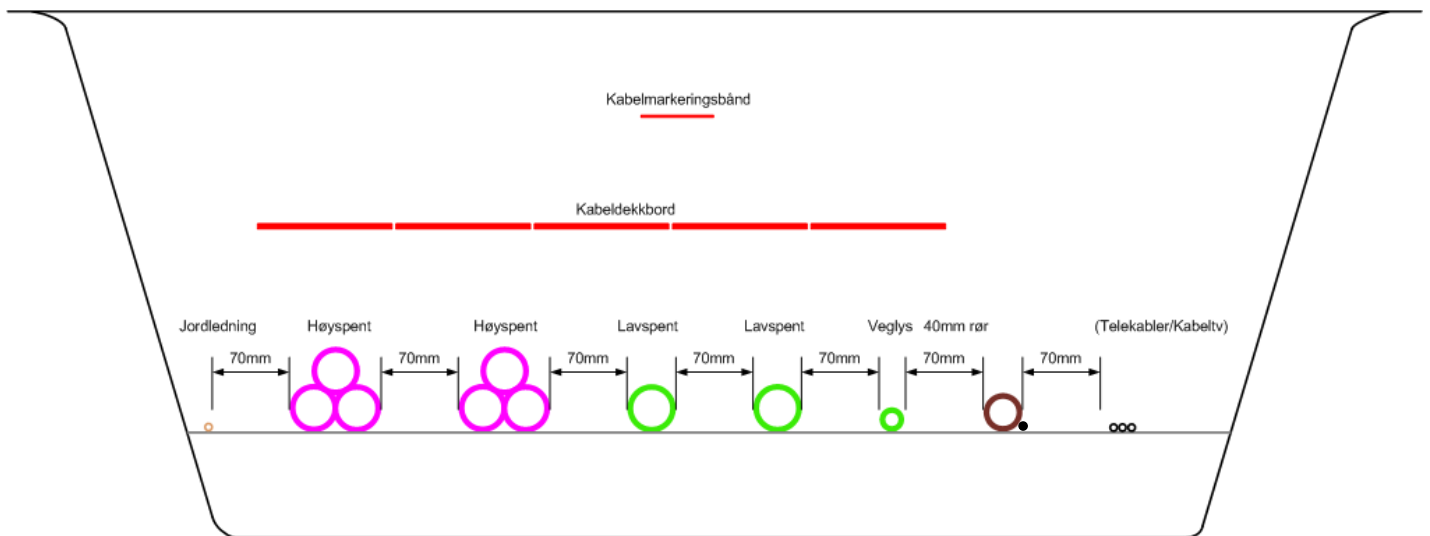
Figur 16. Skisse over kabelplassering i grøften
