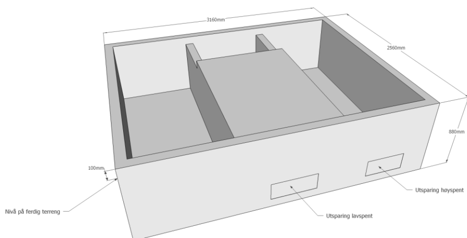
Figur 7. Skisse av betongnettstasjon fundament, Mini-A
