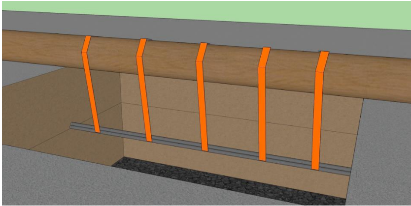
Figur 33. Eksempelløsning med festing av kabel med stropp pr 1 meter.
