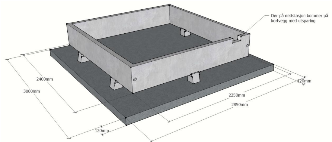
Figur 5. Fundament til prefabrikkert nettstasjon hvor fundamentet er 2400x2250 mm.
