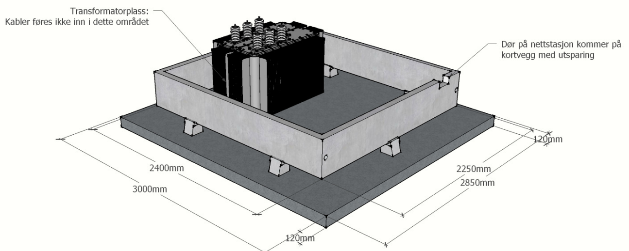
Figur 18. Innføring av kabler i prefabrikkert nettstasjon
