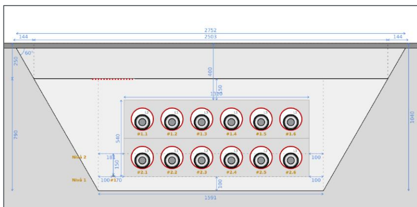
Figur 4-1 Prinsippskisse grøftesnitt omstøpt rørpakke i gang-/sykkelvei
