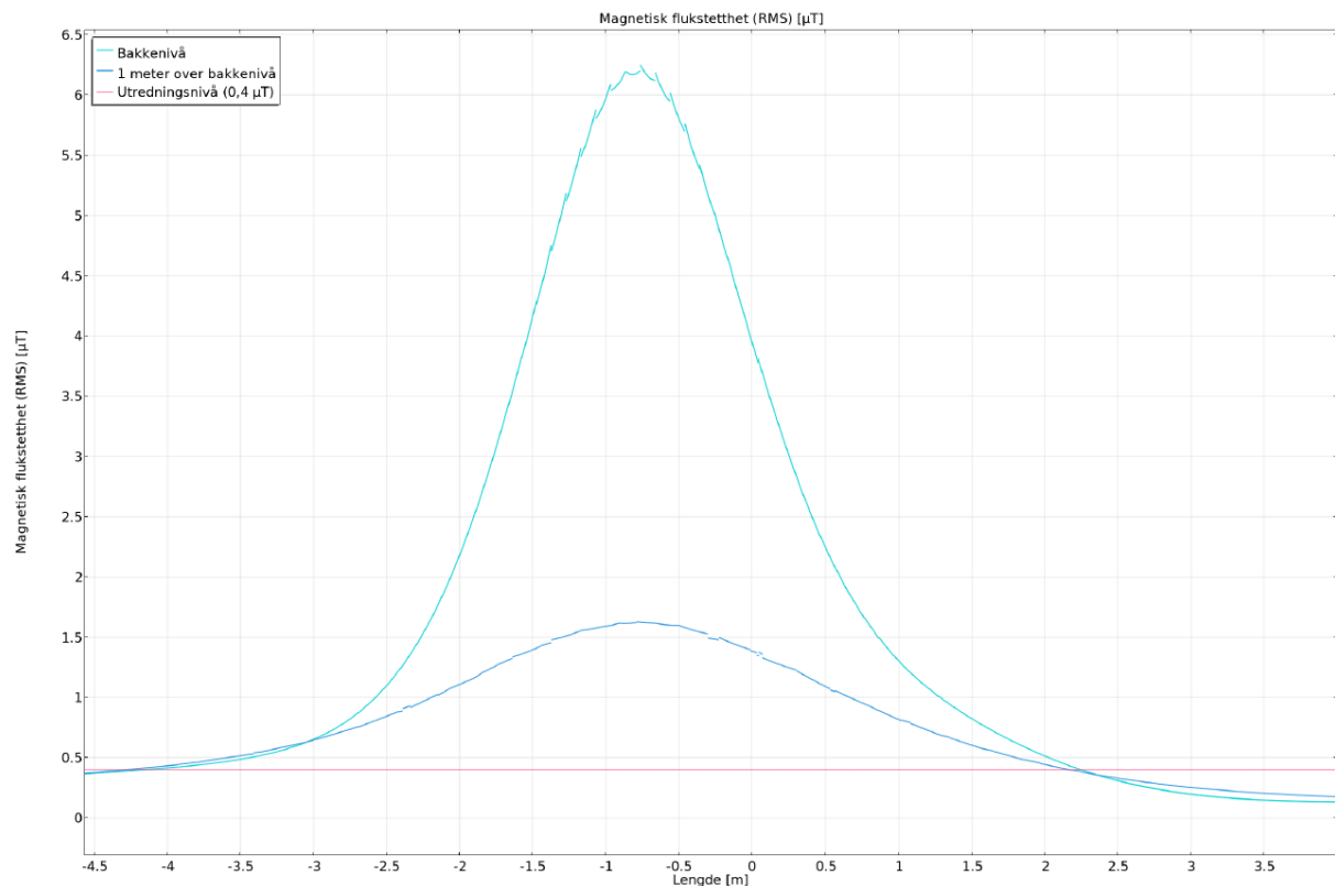
Figuren viser magnetisk flukstetthet [ \mu T ] som RMS-verdier (ikke toppverdier).
