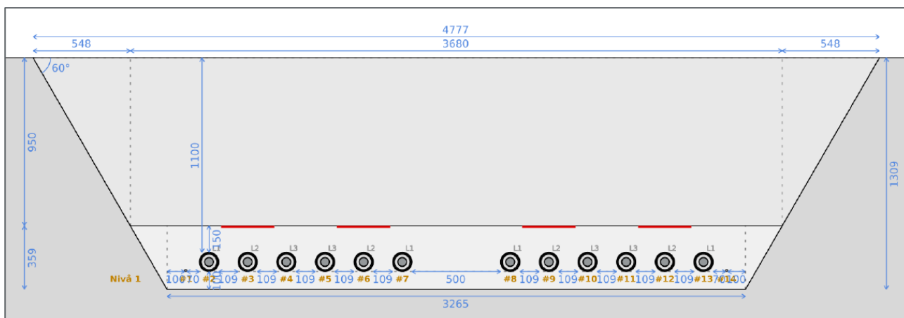
Figur 4-2 Prinsippskisse grøft i ut-/innmark
