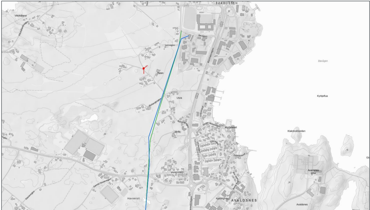
Figur 2-11. Traséalternativ 1 gjennom delområde 1 (markert i blå). Dagens 66 kV-ledning som rives er vist i grønn. Fotostandpunkt for visualisering fra Rehaugane er markert i rødt.
