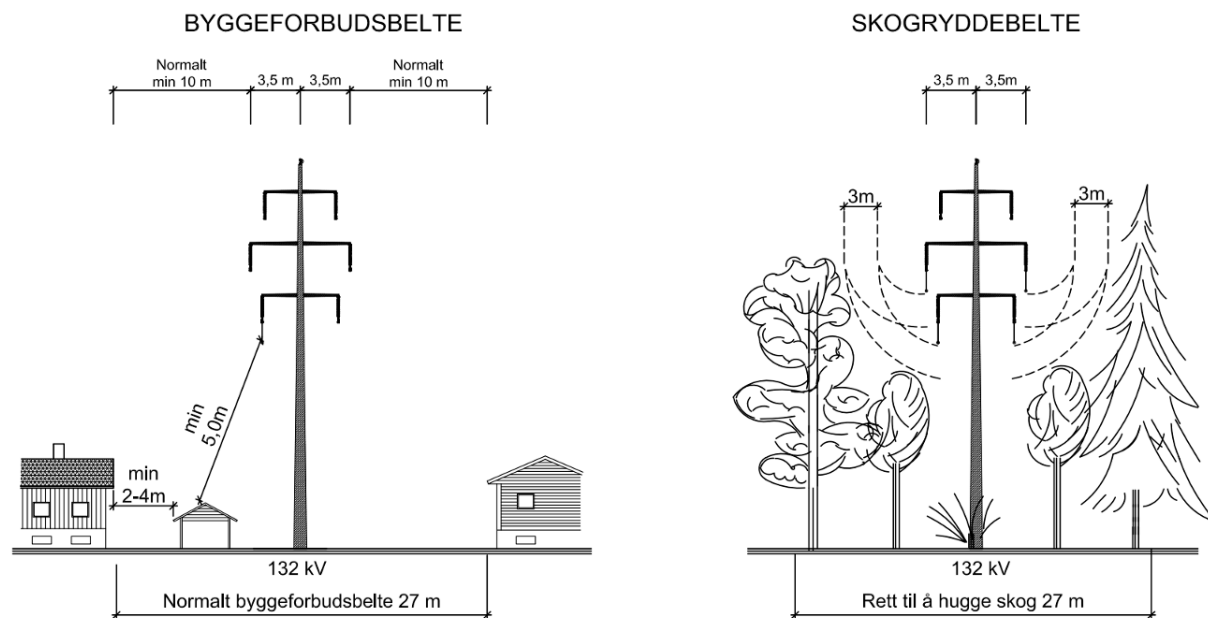
Figur 1-1. Masteskitse av konsekvensutredet dobbeltkurs stålørsmast. Tegning: Jøsok Prosjekt.
